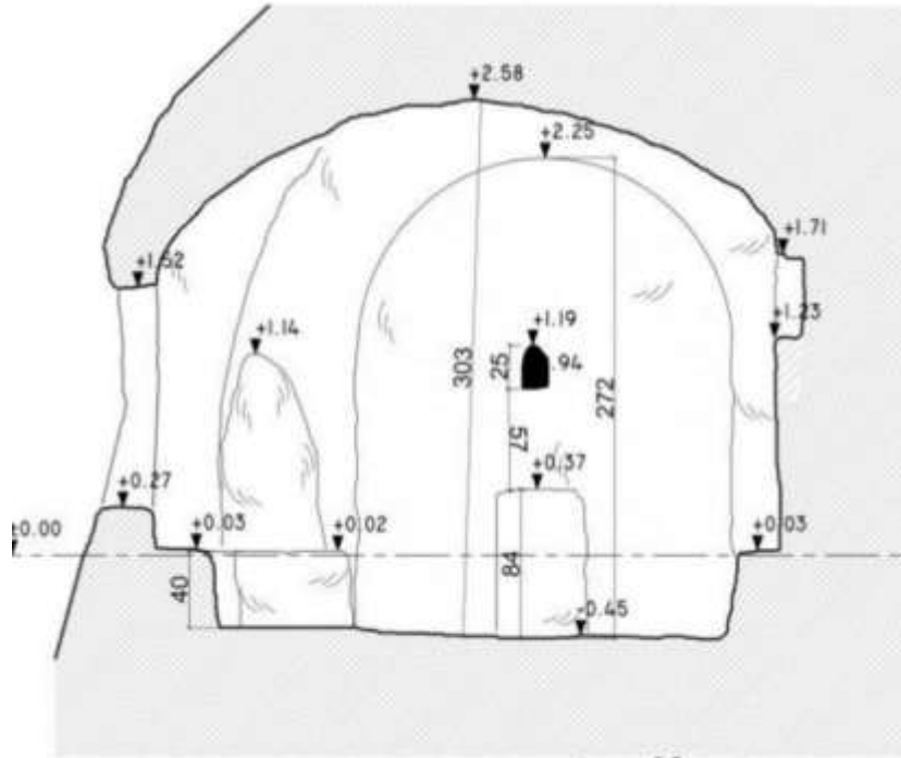
KİLİSTRA İLYASBABA KÖYÜ 1 NOLU ŞAPEL C-C KESİTİ
